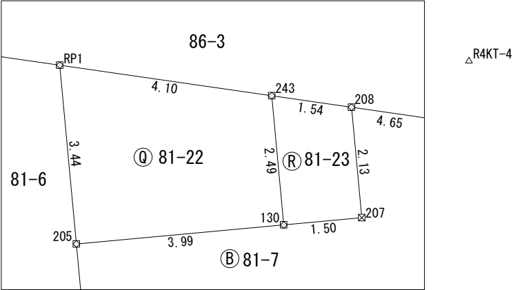
拡大図A 1/100
